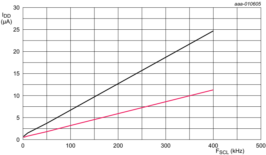
T amb = 25 °C; CLKOUT disabled. (1) V DD = 5.0 V. (2) V DD = 3.3 V.
