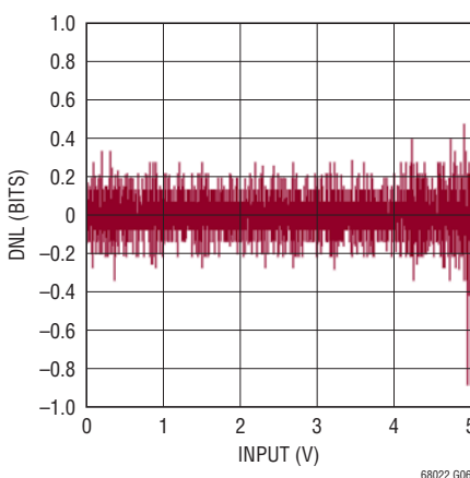
ADC DNL
