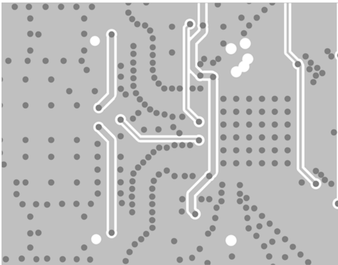
Inner Layer 4
