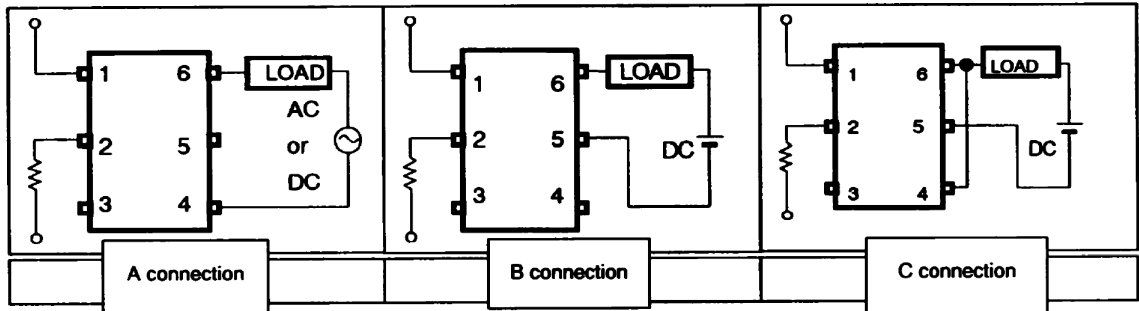
G3VM-355JR, -355JR(TR)
