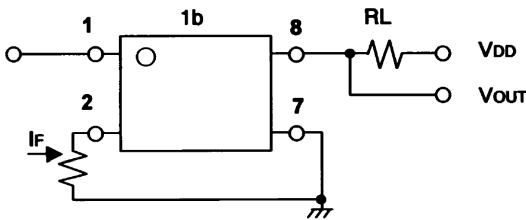
G3VM-355JR, -355JR(TR)
