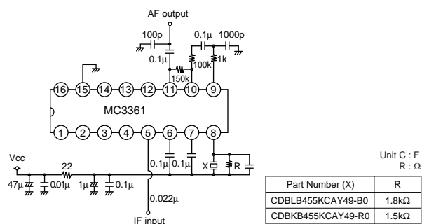
MC3361
