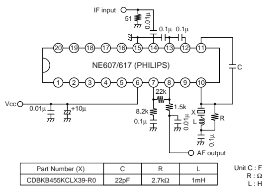
NE(SA)607/617
