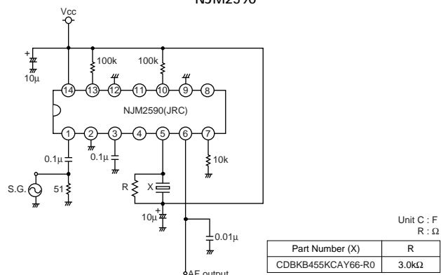
NJM2590
