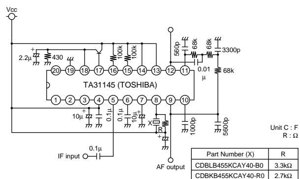
TA31145
