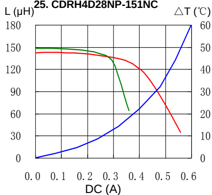
25. CDRH4D28NP-151NC
