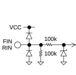
Figure 40. FIN / RIN
