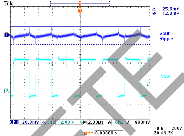
Vout Ripple (VIN = 5V, VOUT = 3.3V, IOUT = 2A)
