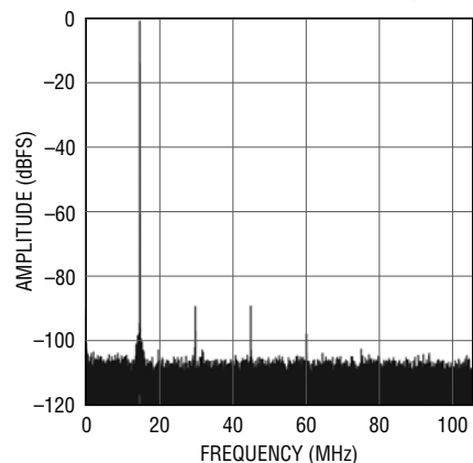
LTC2156-14: 32K Point FFT, f_{IN} = 15\text{MHz} , -1\text{dBFS} , 210\text{Mps}
