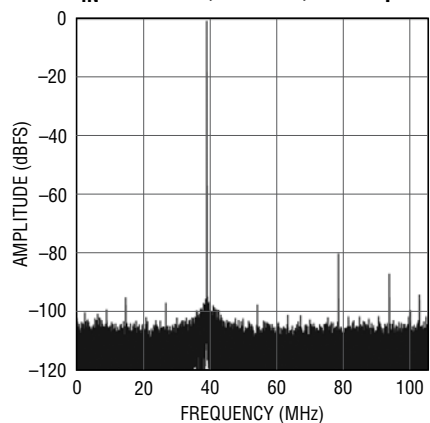
LTC2156-14: 32K Point FFT, f_{IN} = 171\text{MHz} , -1\text{dBFS} , 210\text{Mps}
