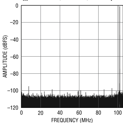
LTC2156-14: 32K Point FFT, f_{IN} = 101\text{MHz} , -1\text{dBFS} , 210\text{Mps}
