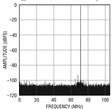
LTC2156-14: 32K Point FFT, f_{IN} = 71\text{MHz} , -1\text{dBFS} , 210\text{Mps}
