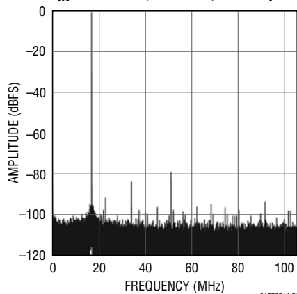
LTC2156-14: 32K Point FFT, f_{IN} = 227\text{MHz} , -1\text{dBFS} , 210\text{Mps}
