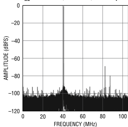
LTC2156-14: 32K Point FFT, f_{IN} = 379\text{MHz} , -1\text{dBFS} , 210\text{Mps}
