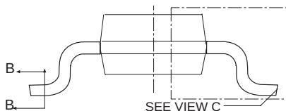
VIEW A-A
