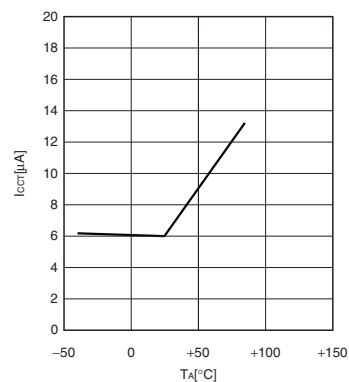
I_{CCTS} - T_A
