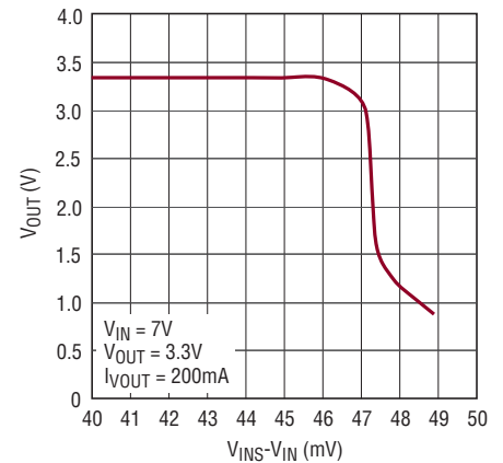
VOUT vs VINS-VIN
