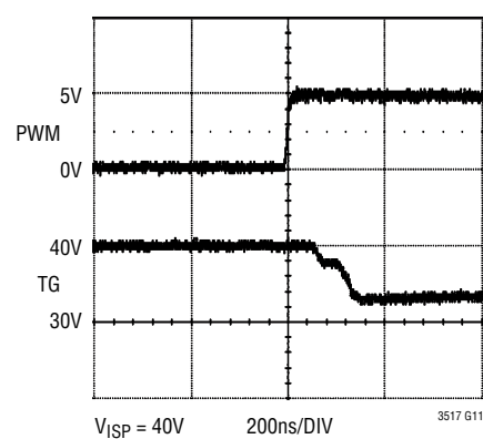
PMOS Turn-On
