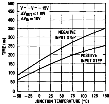
Aperture Time*
