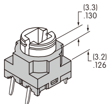
Extended Actuator
