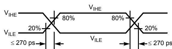
(d) CML/LVPECL Input Test Waveform
