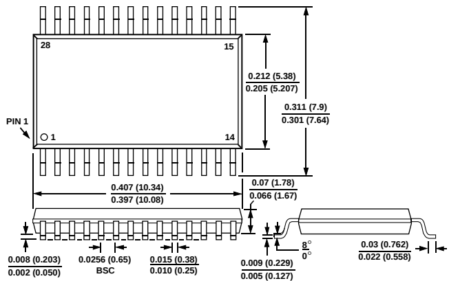
SSOP (RS-28)
