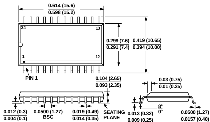
SOIC (R-24)
