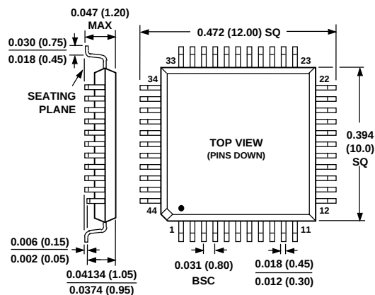
TQFP (SU-44)
