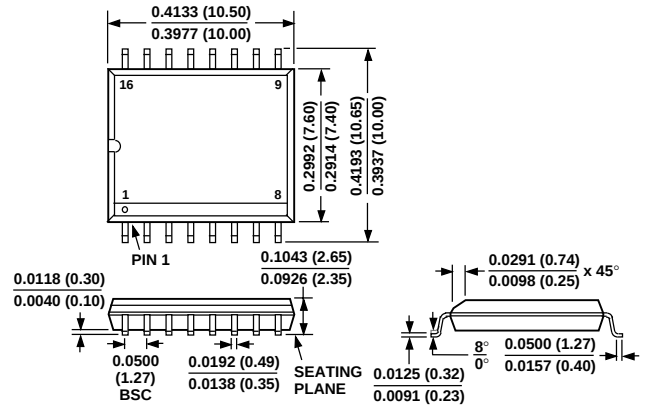
SOIC (R-16)
