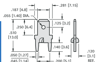
.187 (4.8) TAB
