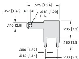
.110 (2.8) TAB
