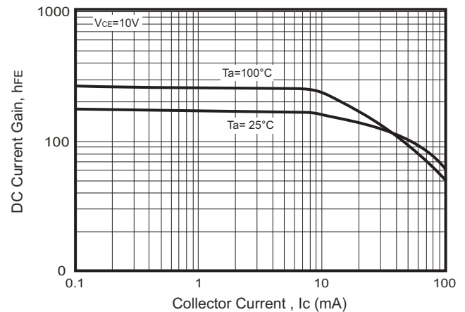
Fig.2 - h_{FE} - I_c
