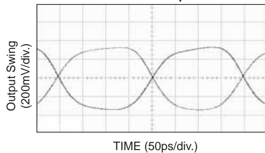
2.5GHz Output
