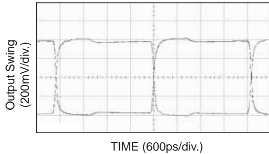
200MHz Output
