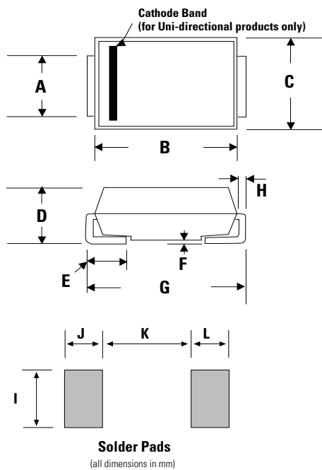
DO-214AA (SMB J-Bend)
